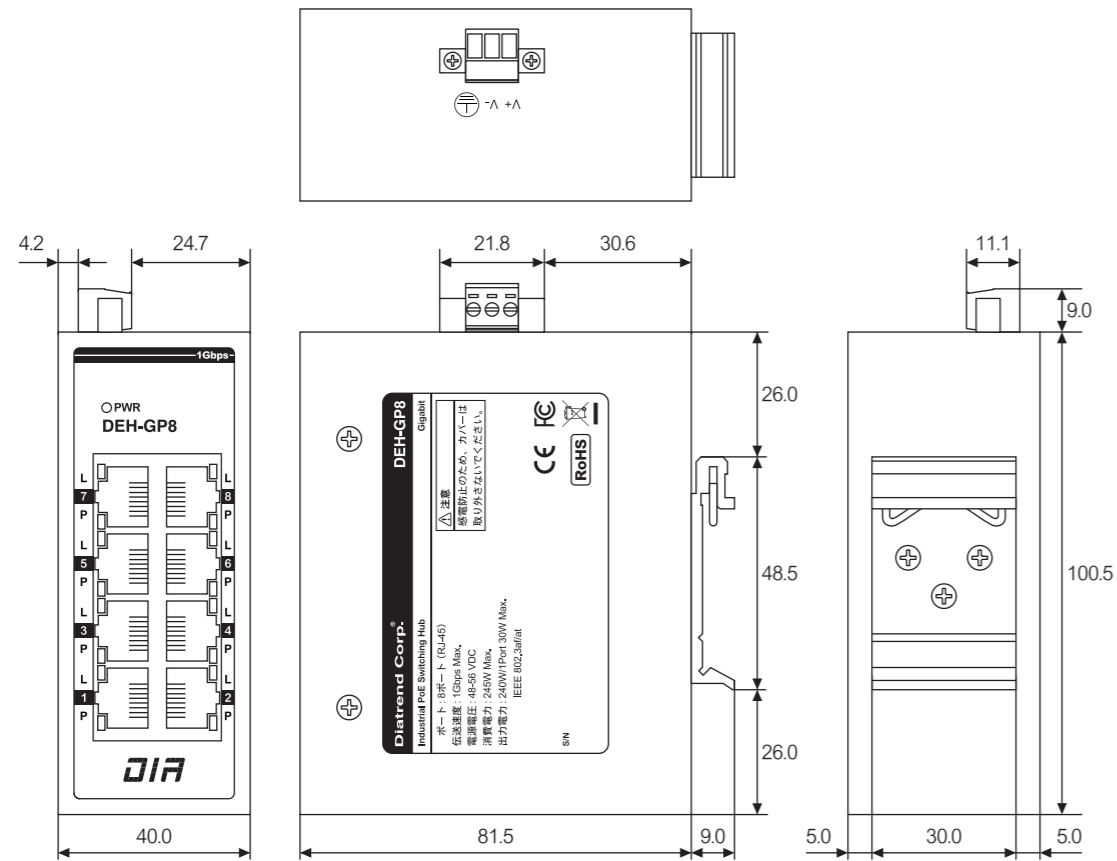
単位 : mm
